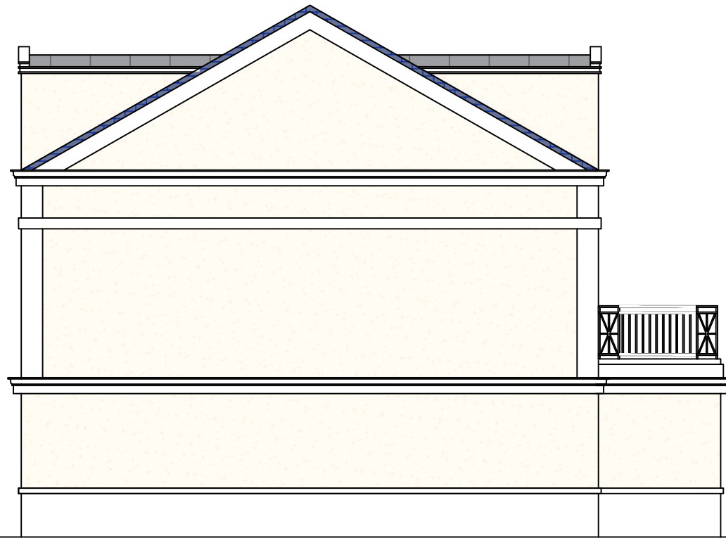
Façade Nord
